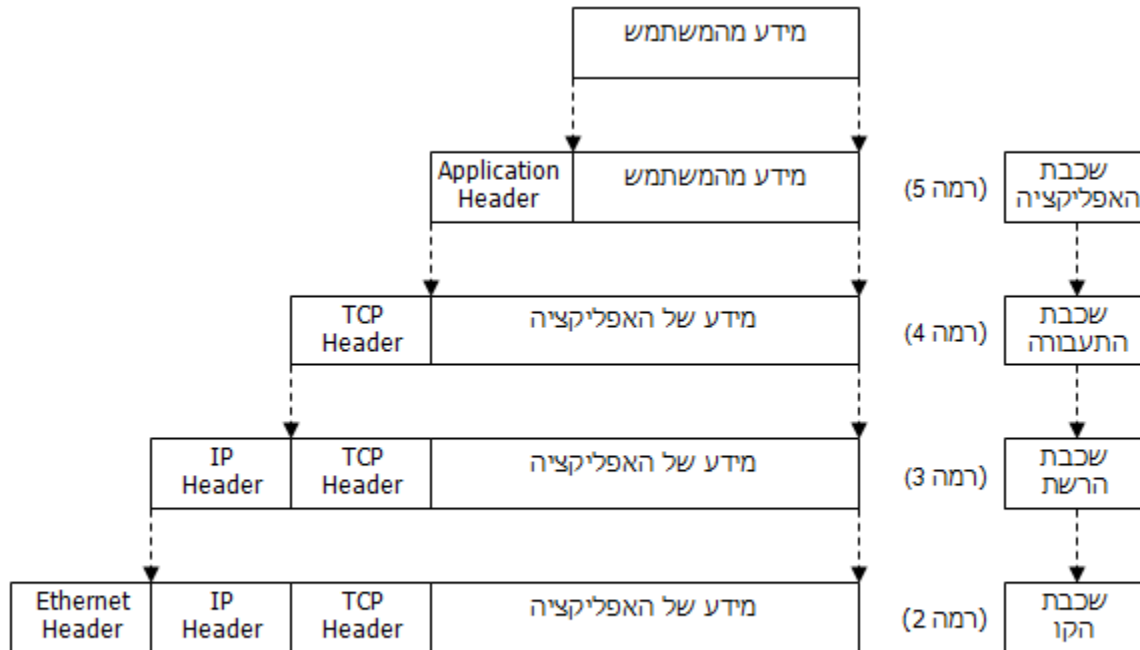
מבנה פקטה במודל חמש השכבות 2#
